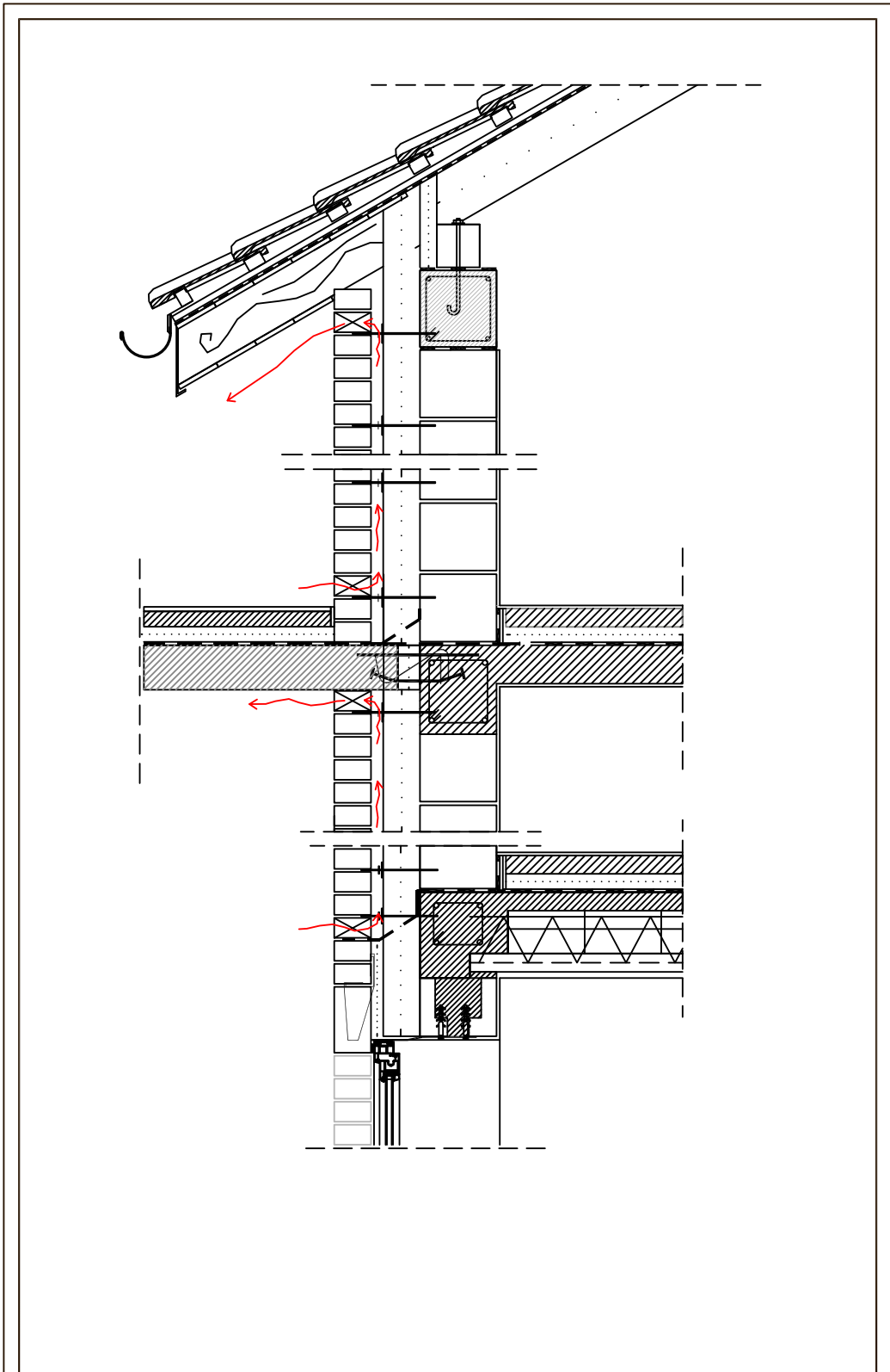
Rys B1 WENTYLACJA W ŚCIANIE TRÓJWARSTWOWEJ szczegół usytuowania szczelin wentylacyjnych - strefa poddasza SKALA 1:20
