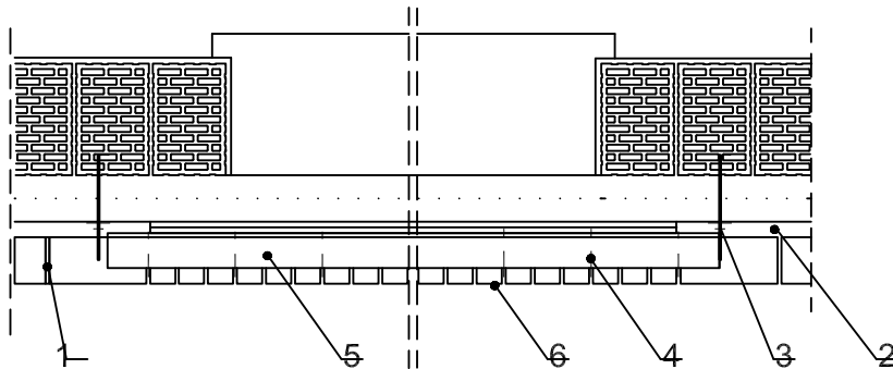
Przekrój A-A
